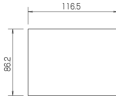
パネルカット寸法
