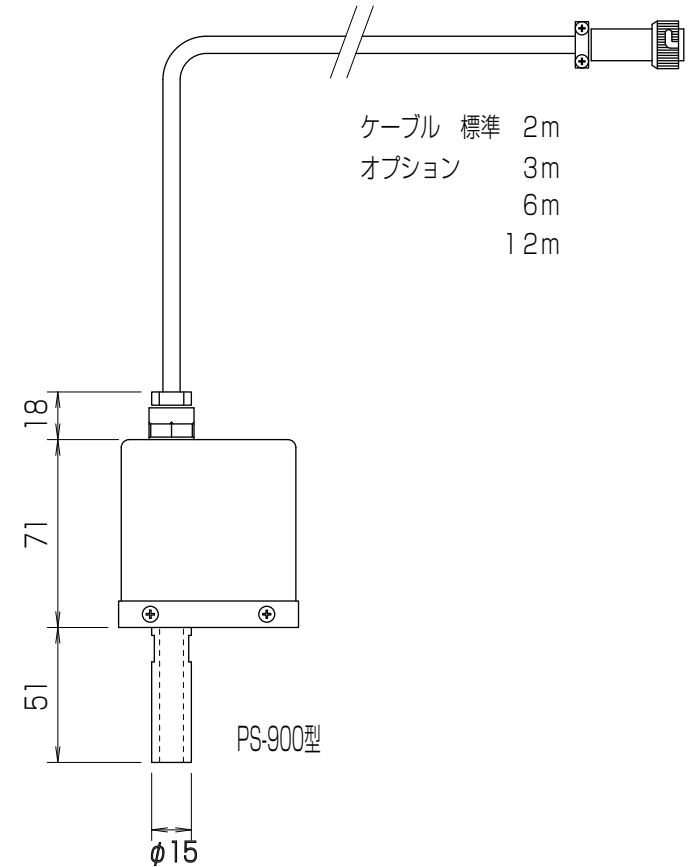
測定子・ケーブル
