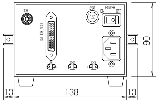
後面図
