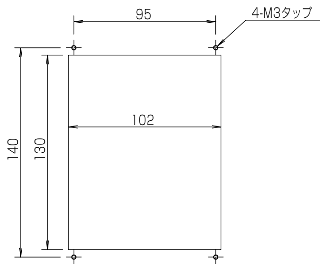
パネルカット寸法
