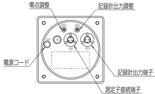
後面図
