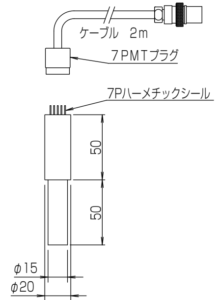
測定子・ケーブル
