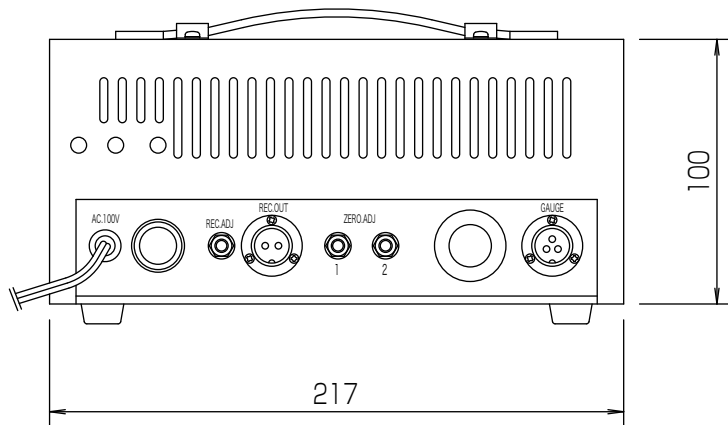
後面図
