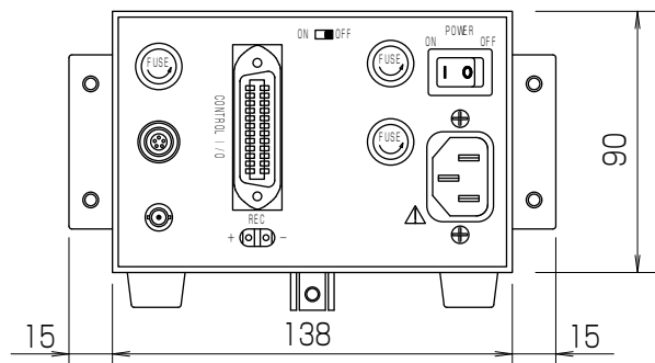
後面図
