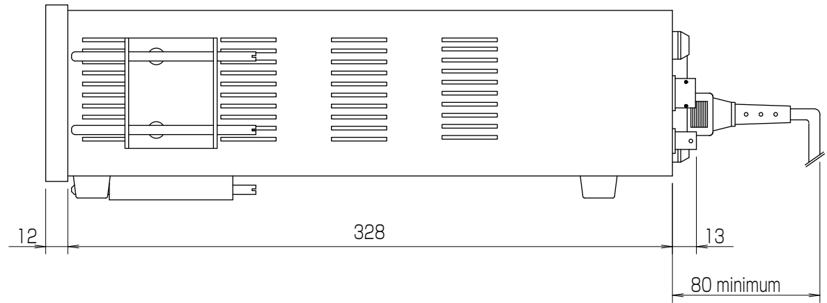
側面図
