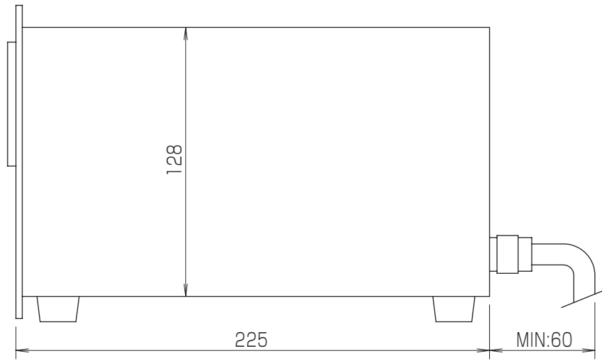
側面図
