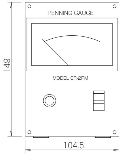
正面図
