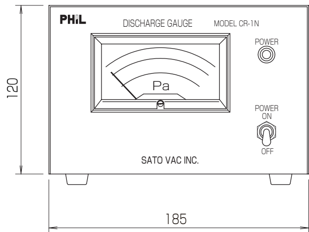
正面図
